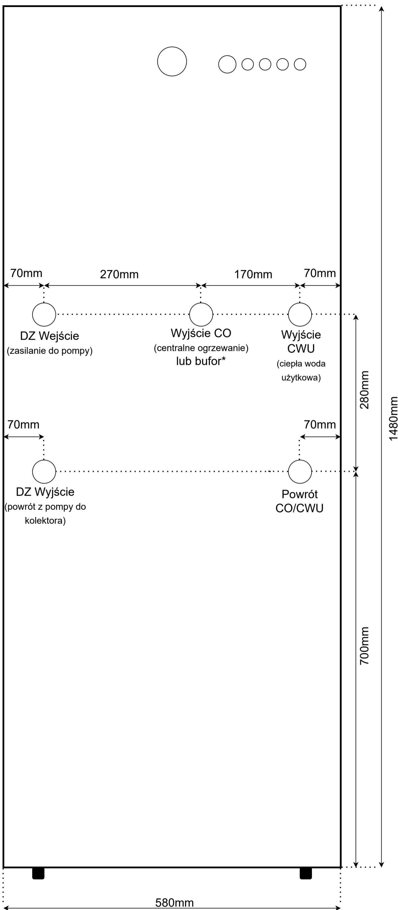
Schemat i wymiary pompy ciepła PPC Ecopower seria C. Widok z tyłu urządzenia.
